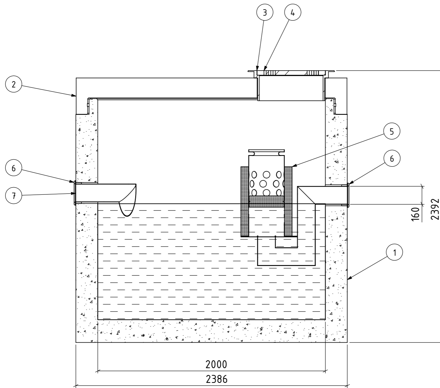
KESKILINJAN LEIKKAUS
