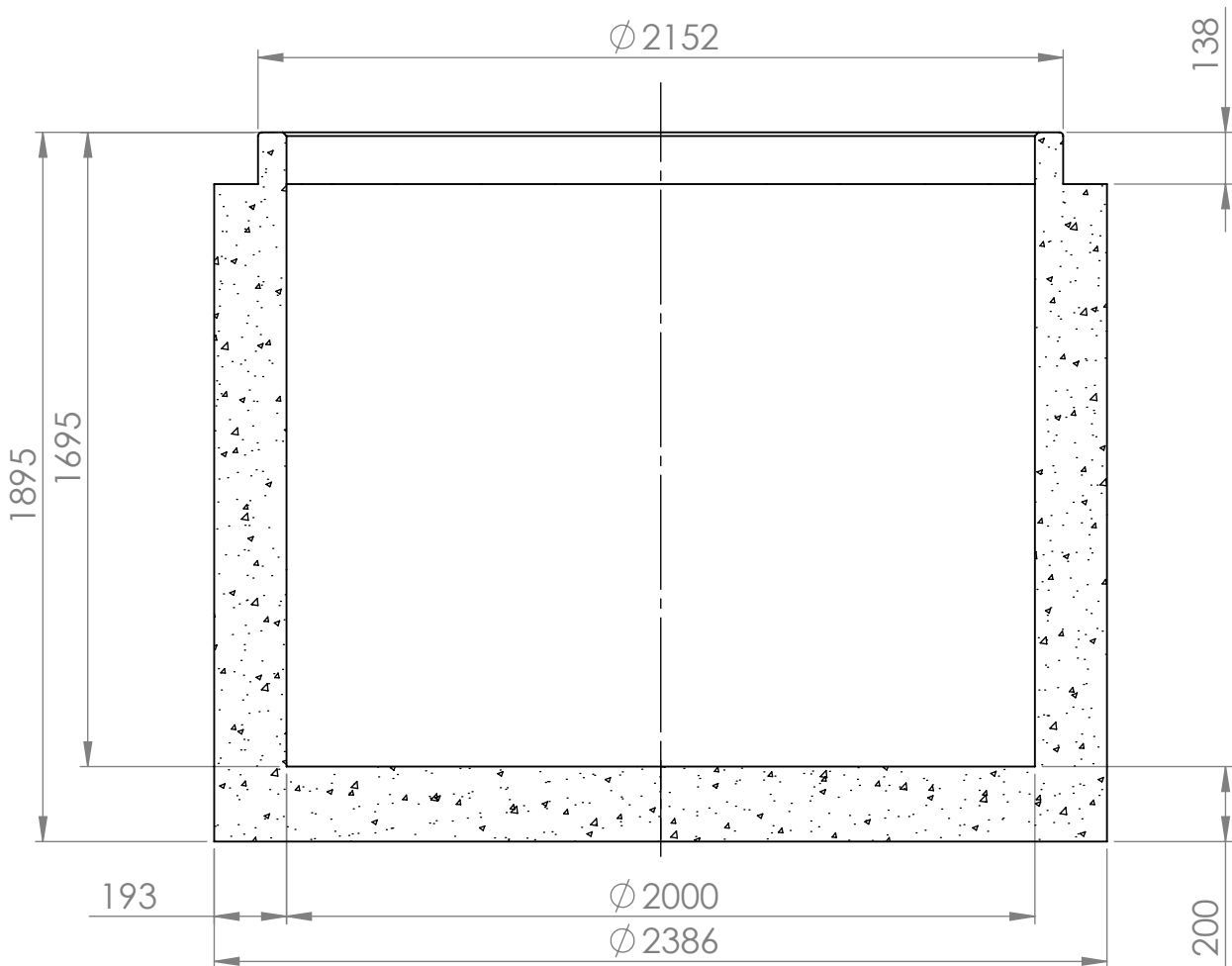
KESKILINJAN LEIKKAUS
