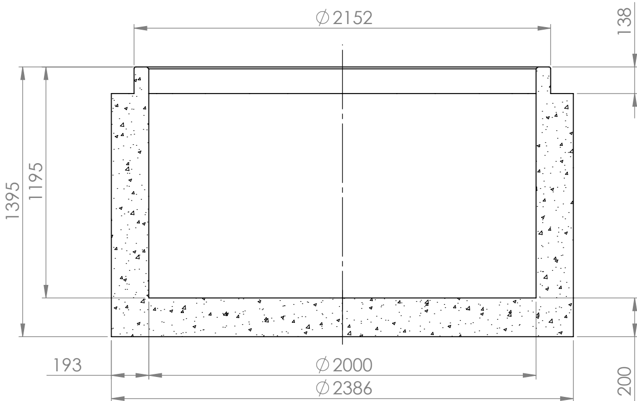
KESKILINJAN LEIKKAUS
