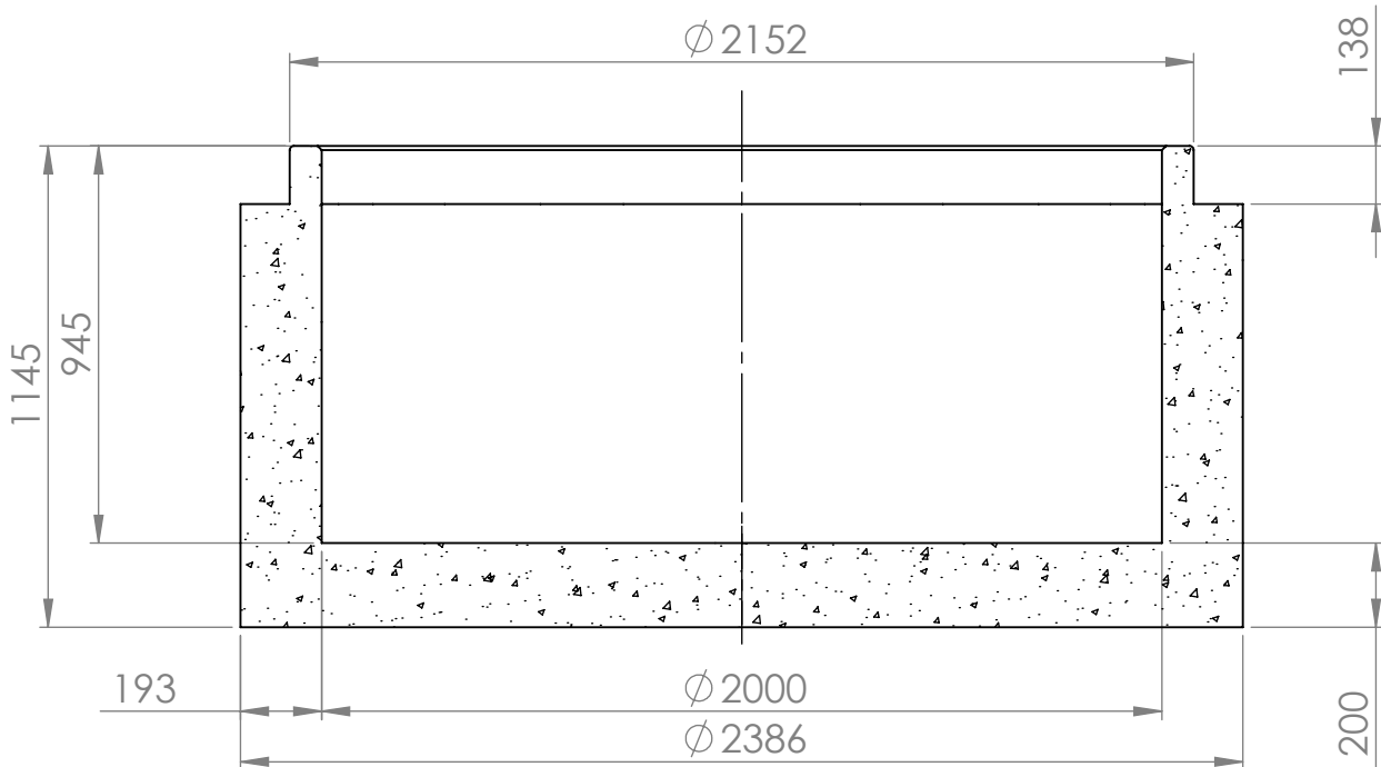
KESKILINJAN LEIKKAUS
