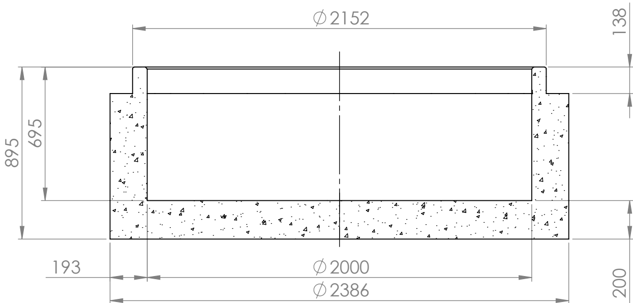
KESKILINJAN LEIKKAUS
