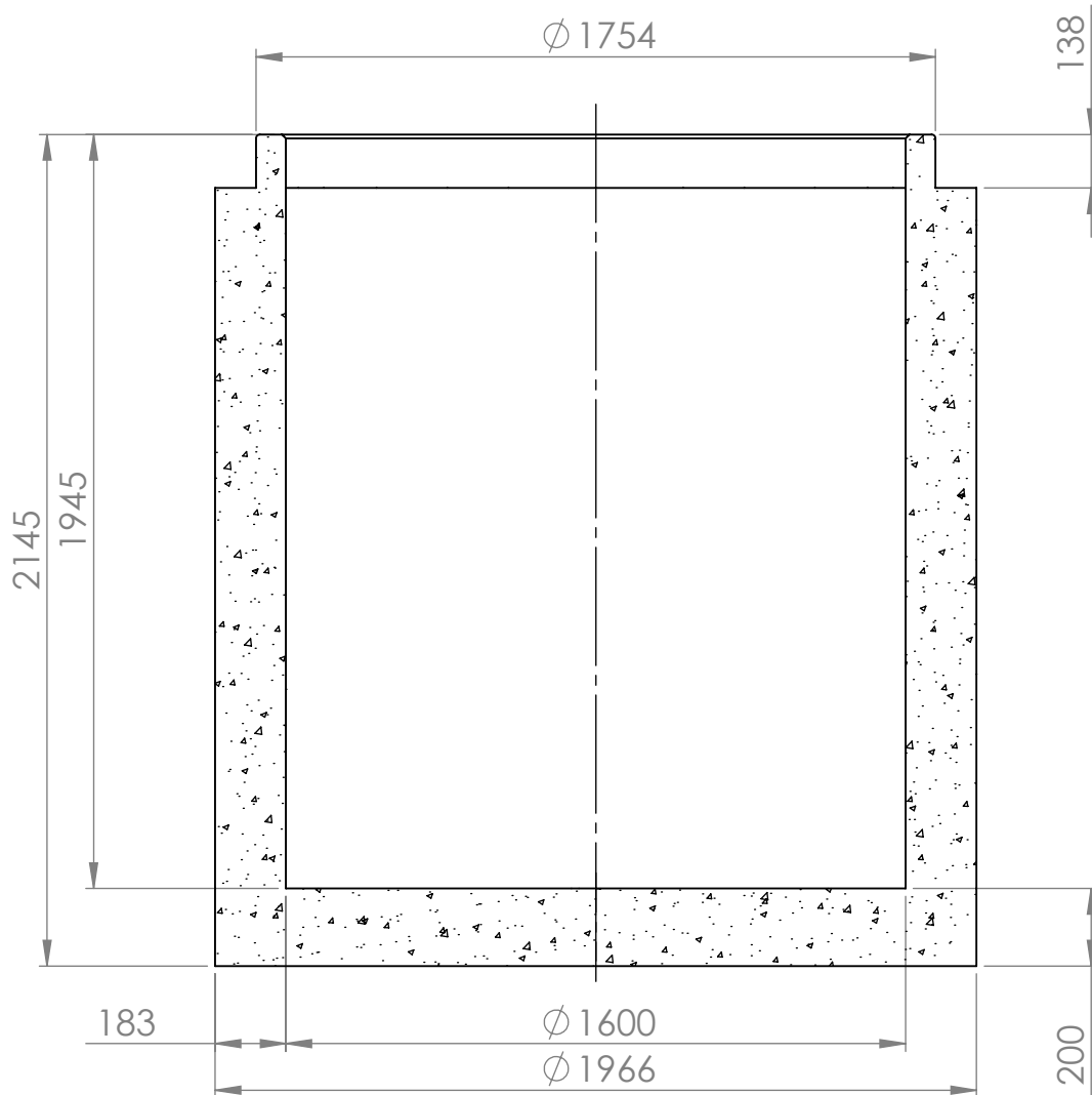
KESKILINJAN LEIKKAUS
