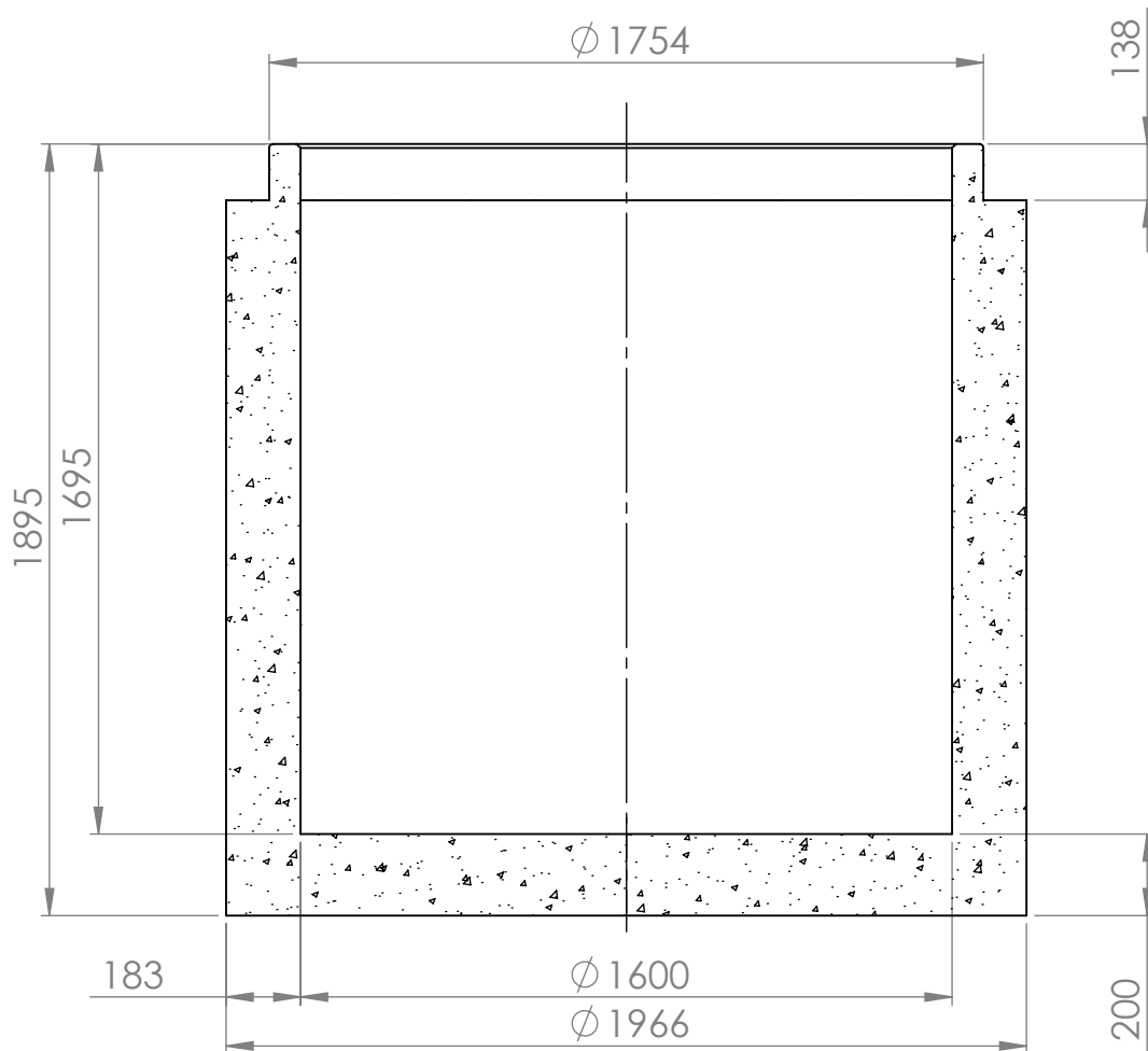
KESKILINJAN LEIKKAUS
