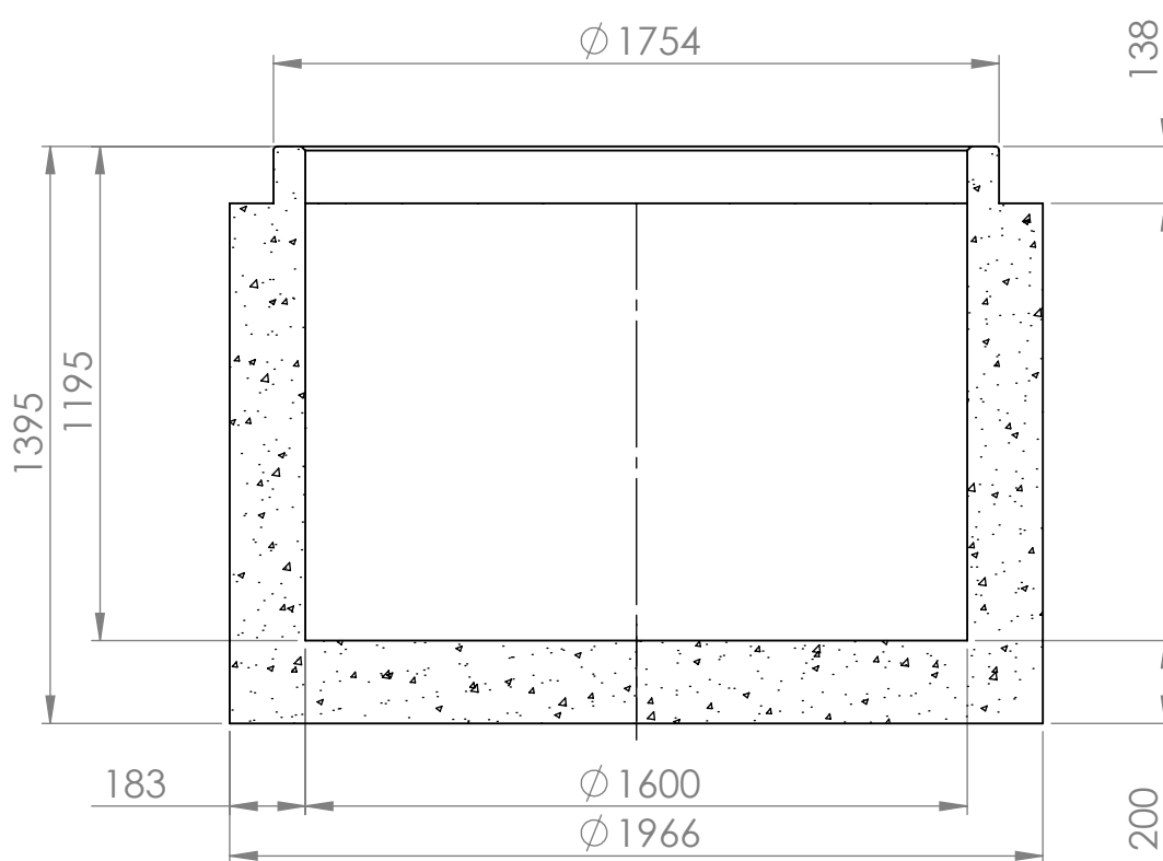
KESKILINJAN LEIKKAUS
