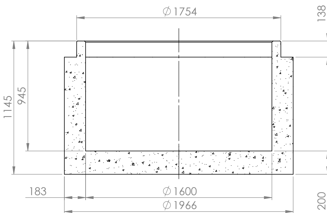
KESKILINJAN LEIKKAUS
