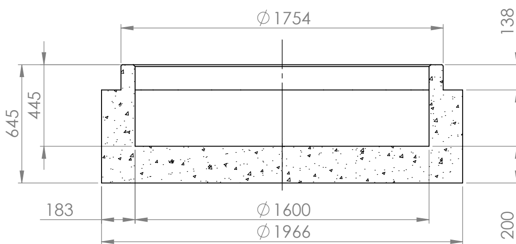
KESKILINJAN LEIKKAUS
