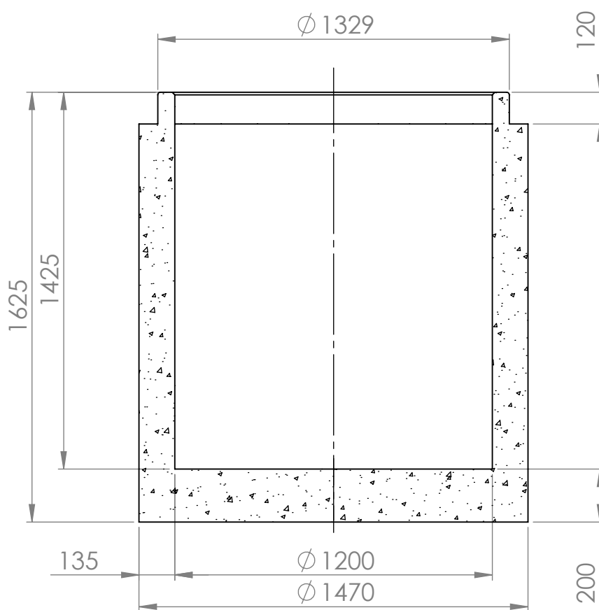
KESKILINJAN LEIKKAUS
