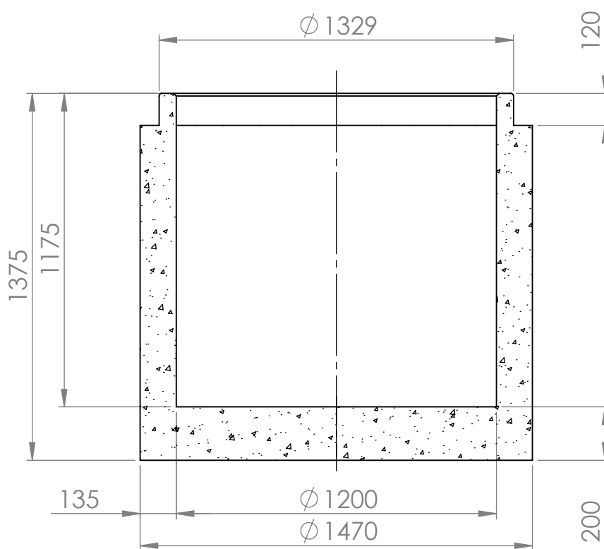
KESKILINJAN LEIKKAUS
