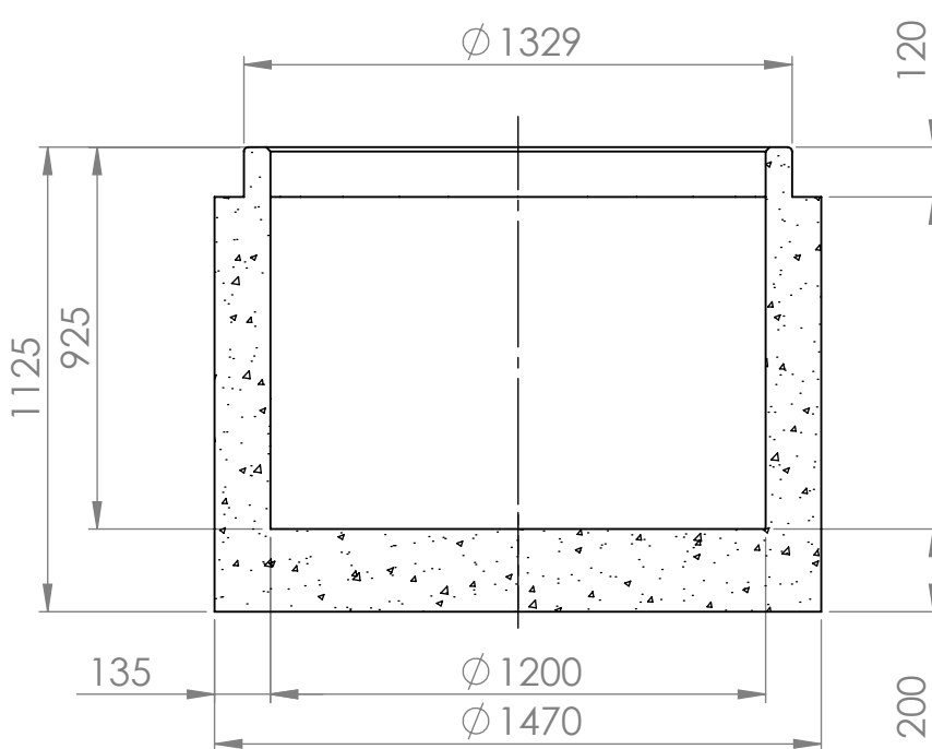
KESKILINJAN LEIKKAUS
