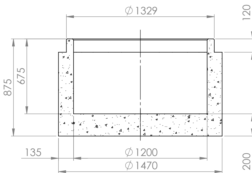
KESKILINJAN LEIKKAUS
