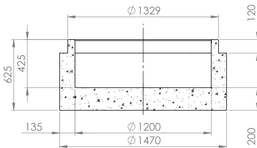
KESKILINJAN LEIKKAUS
