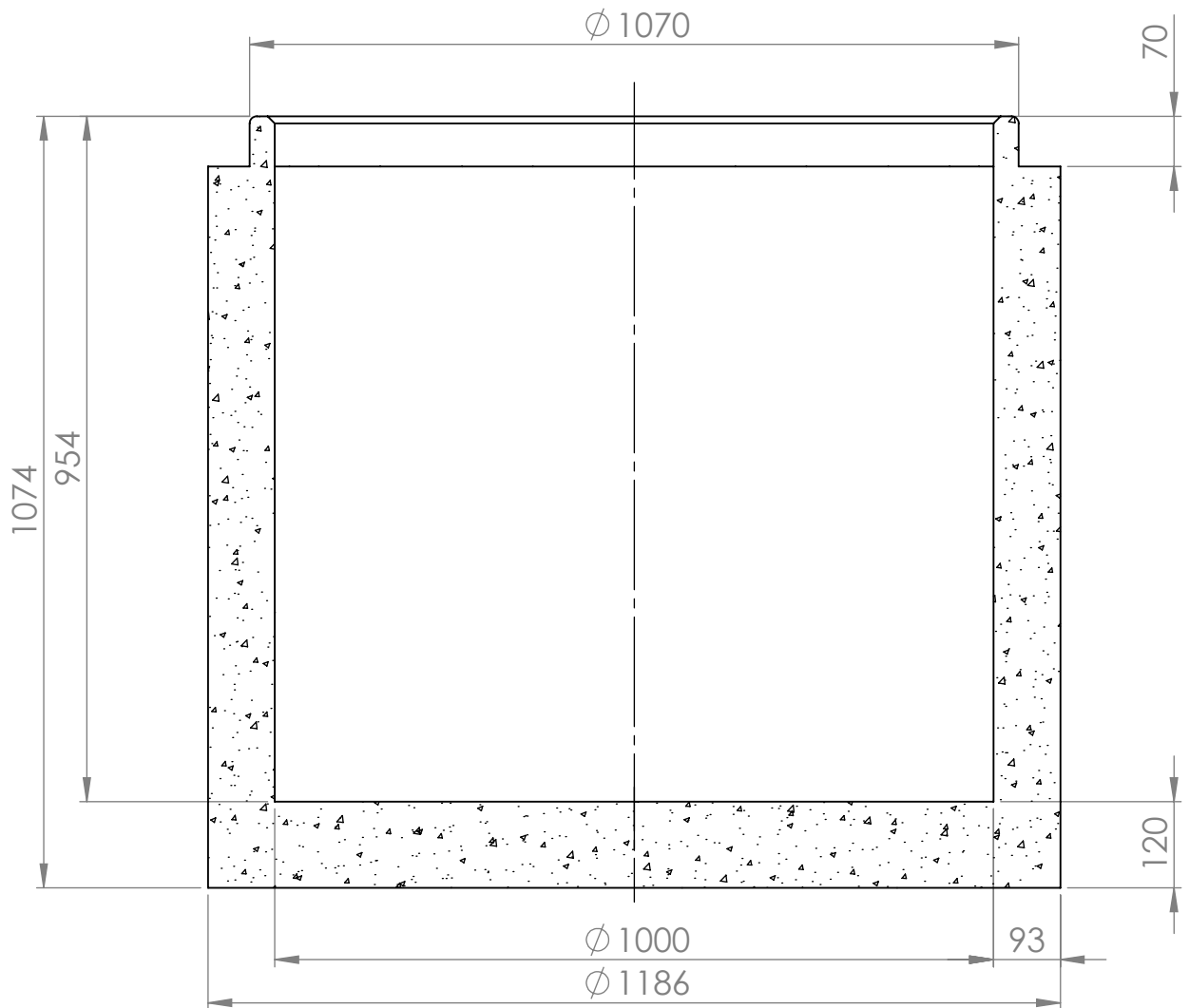
KESKILINJAN LEIKKAUS
