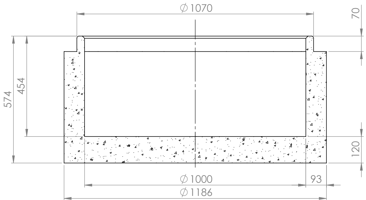
KESKILINJAN LEIKKAUS
