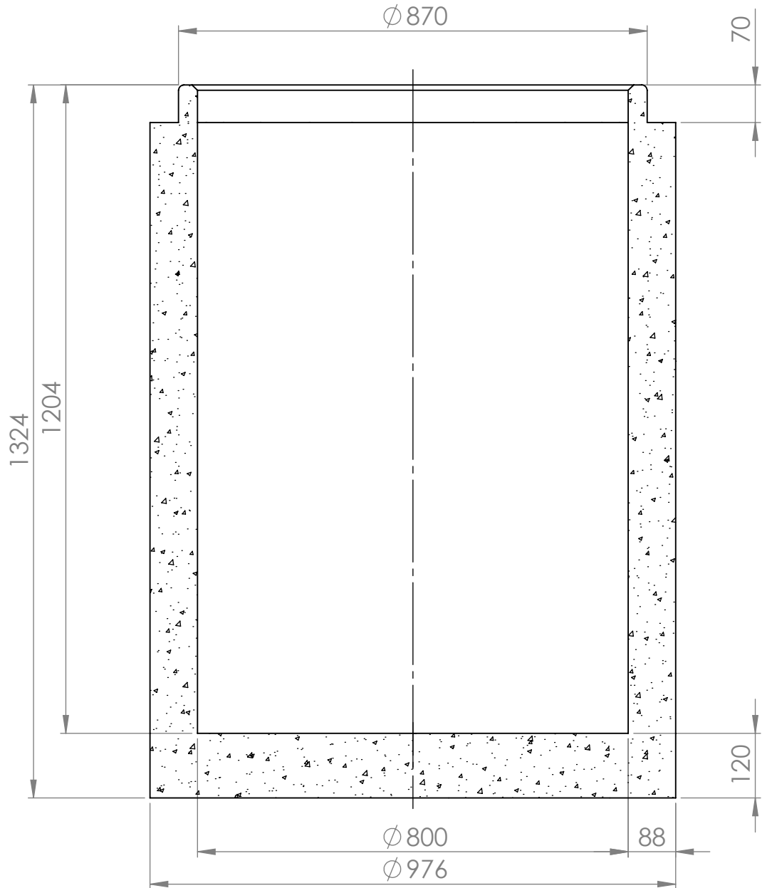
KESKILINJAN LEIKKAUS
