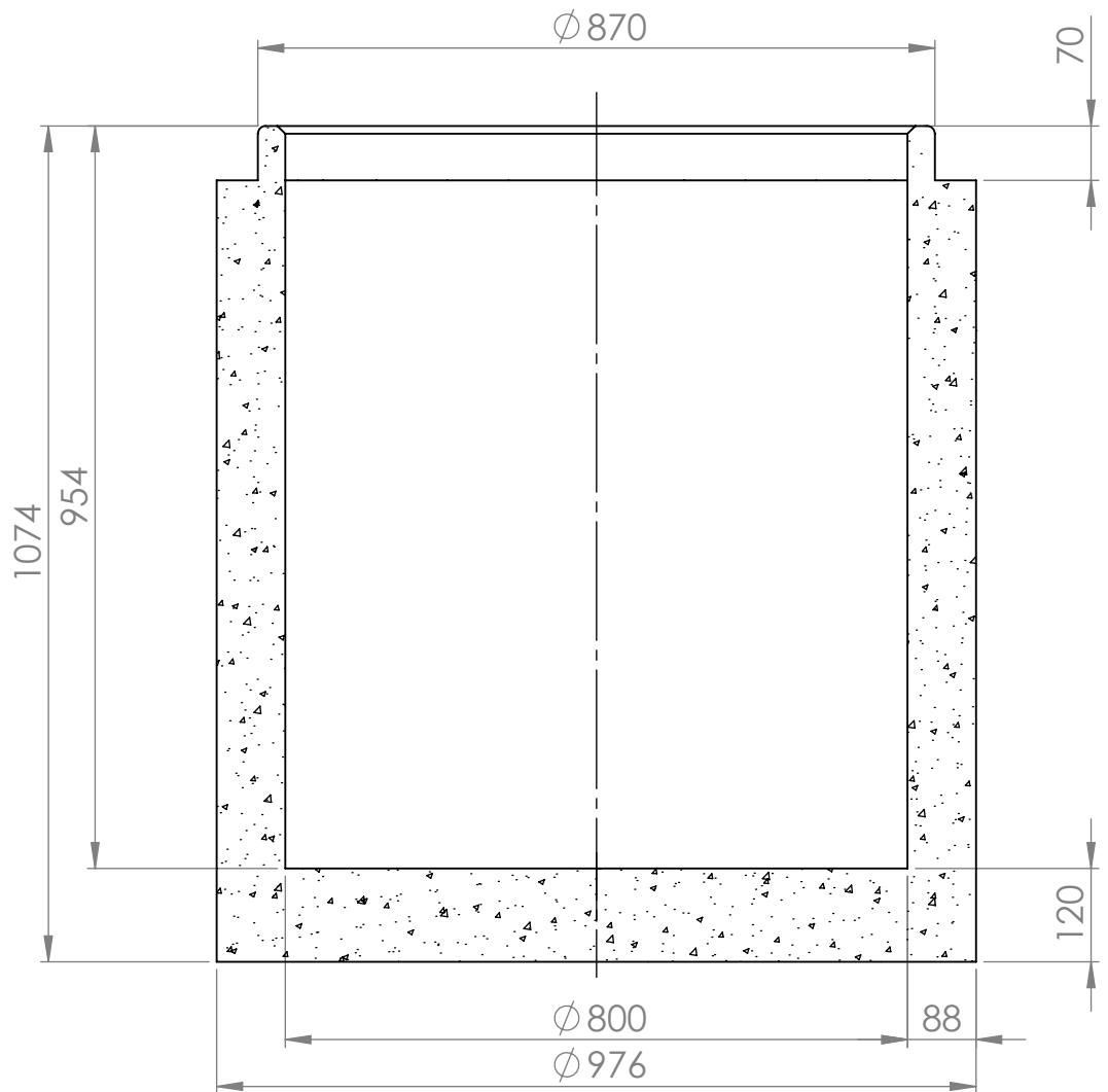
KESKILINJAN LEIKKAUS
