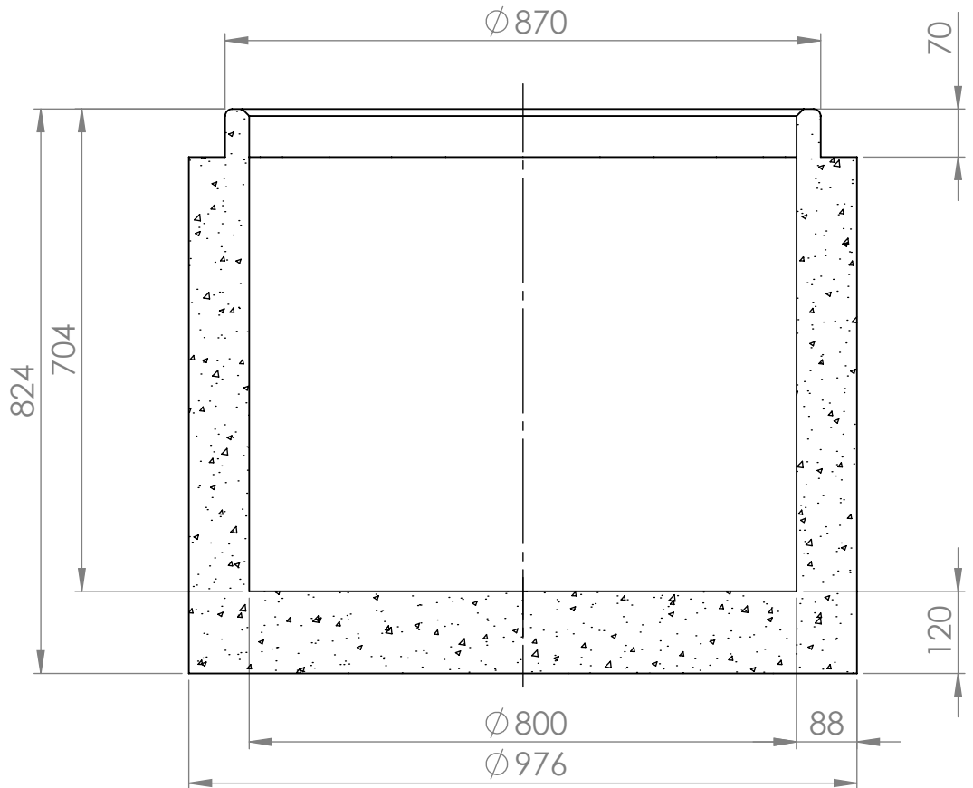
KESKILINJAN LEIKKAUS
