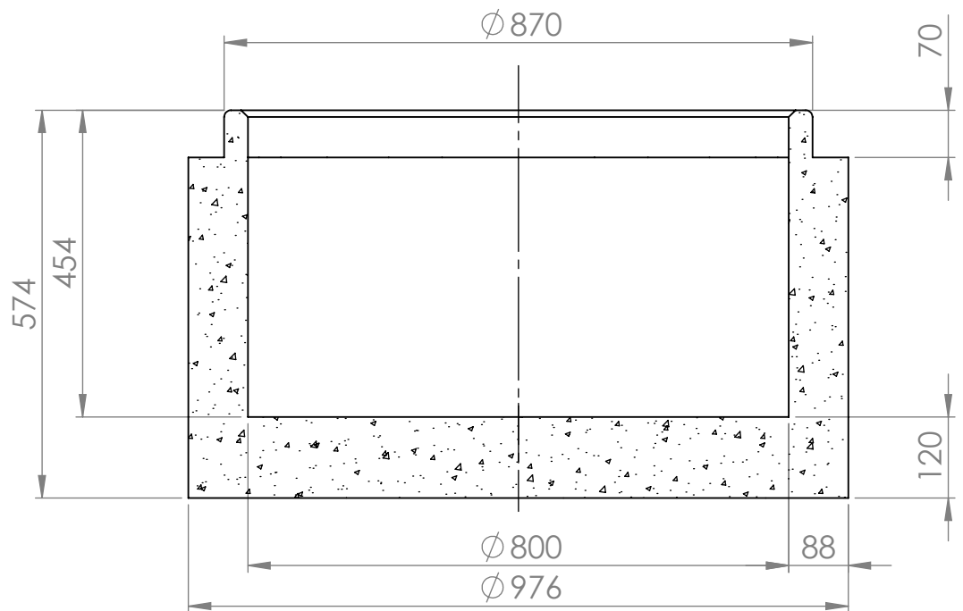
KESKILINJAN LEIKKAUS
