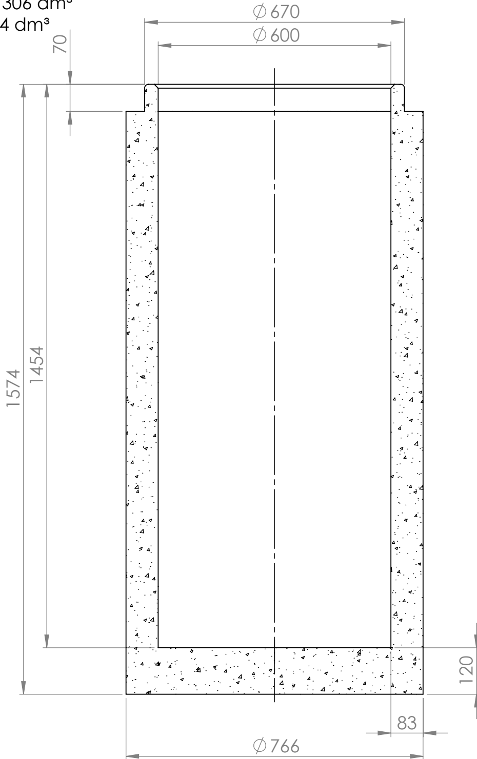
KESKILINJAN LEIKKAUS
