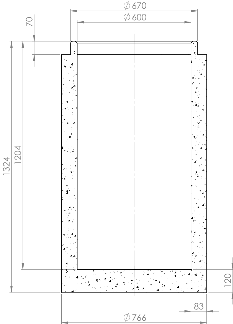
KESKILINJAN LEIKKAUS
