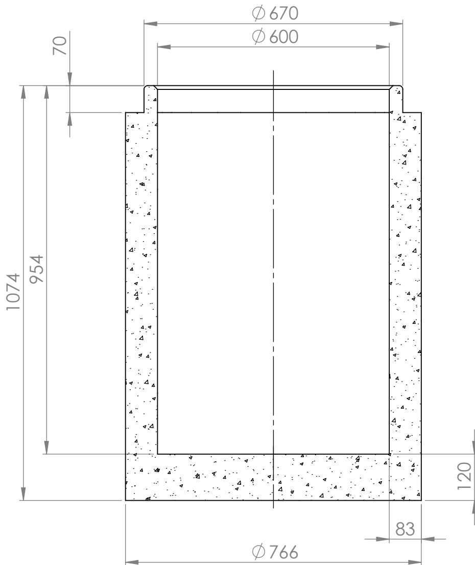
KESKILINJAN LEIKKAUS
