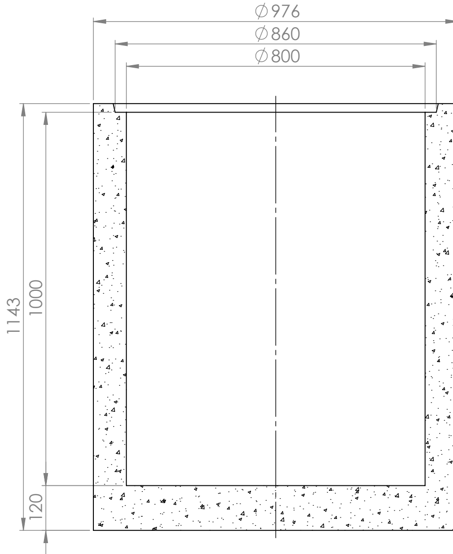
KESKILINJAN LEIKKAUS
