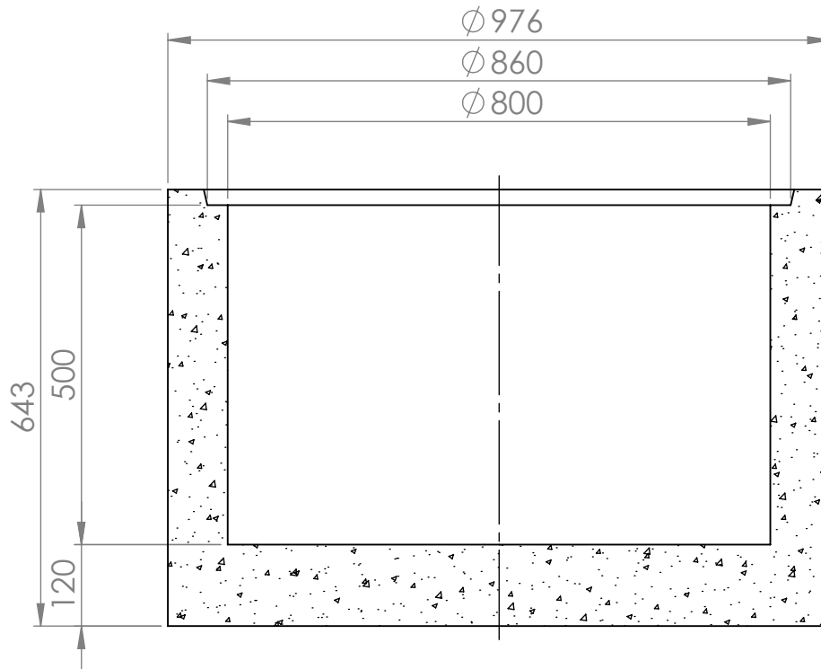
KESKILINJAN LEIKKAUS
