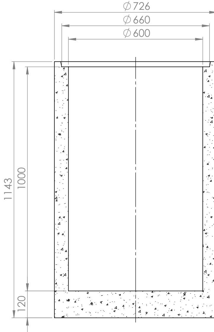
KESKILINJAN LEIKKAUS
