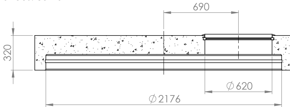
LEIKKAUS A-A
