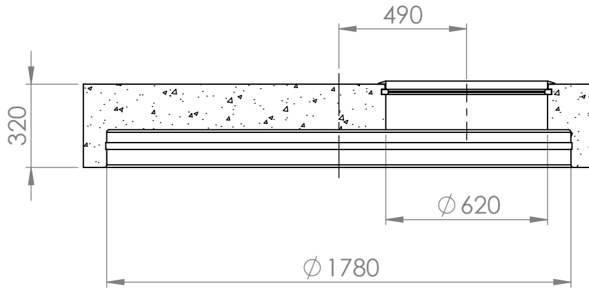
LEIKKAUS A-A
