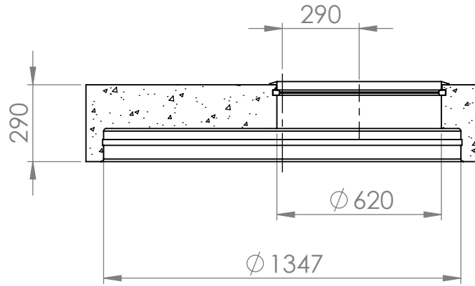
LEIKKAUS A-A
