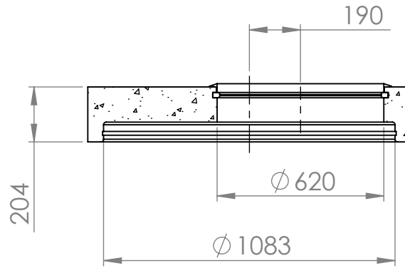
LEIKKAUS A-A
