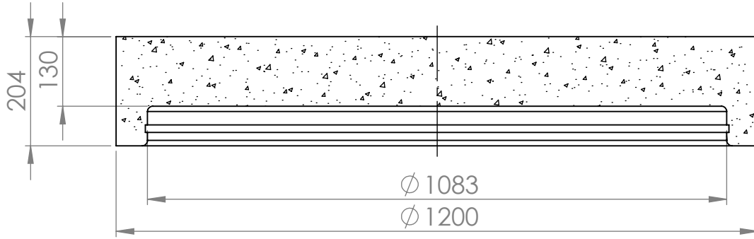
LEIKKAUS A-A
