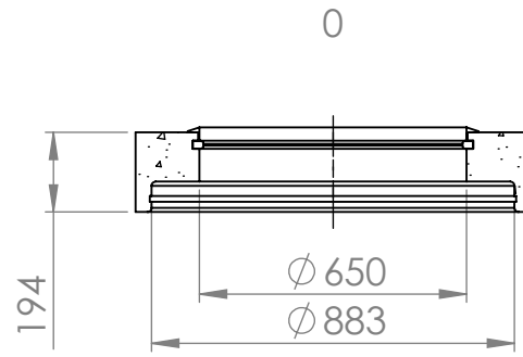
LEIKKAUS A-A
