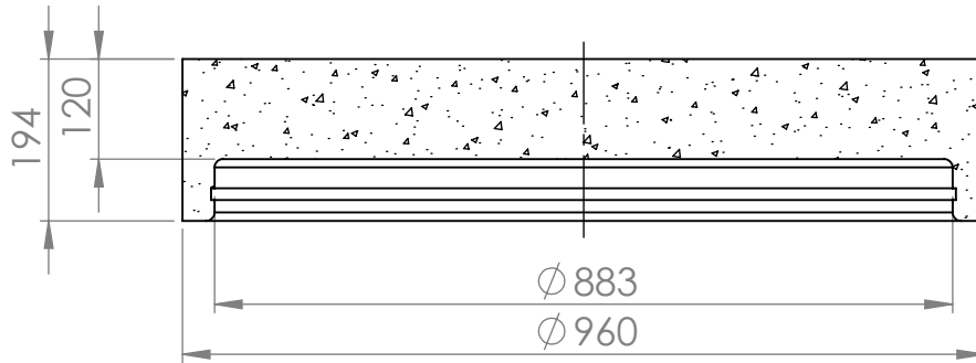
LEIKKAUS A-A
