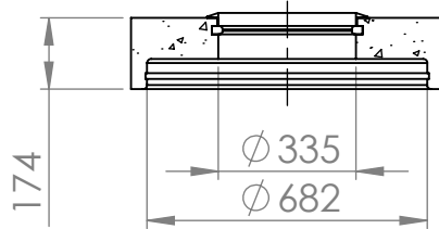
LEIKKAUS A-A
