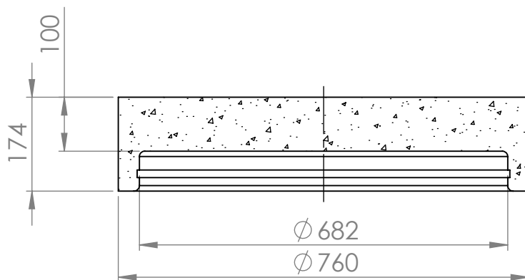
LEIKKAUS A-A
