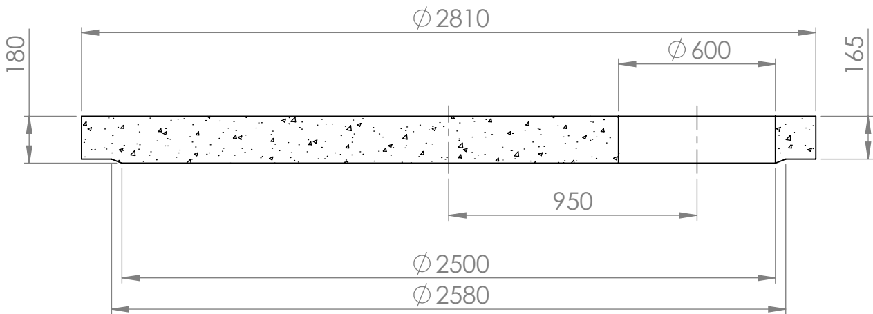
KESKILINJAN LEIKKAUS
