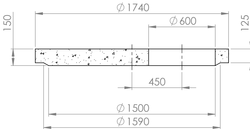
KESKILINJAN LEIKKAUS
