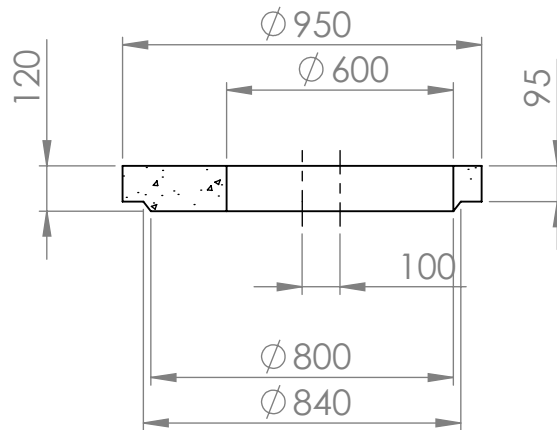
KESKILINJAN LEIKKAUS
