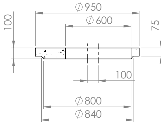
KESKILINJAN LEIKKAUS
