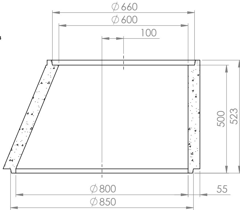
LEIKKAUS A-A
