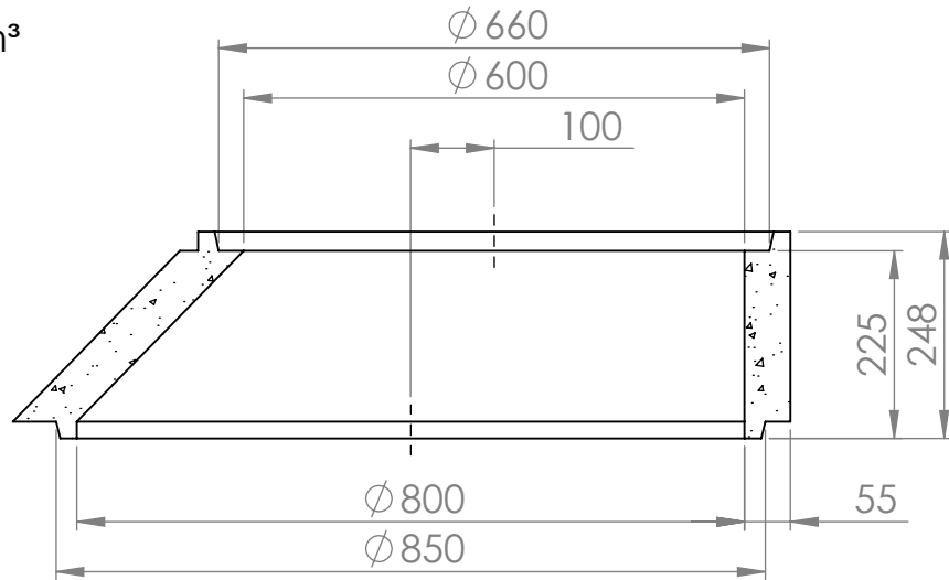
LEIKKAUS A-A
