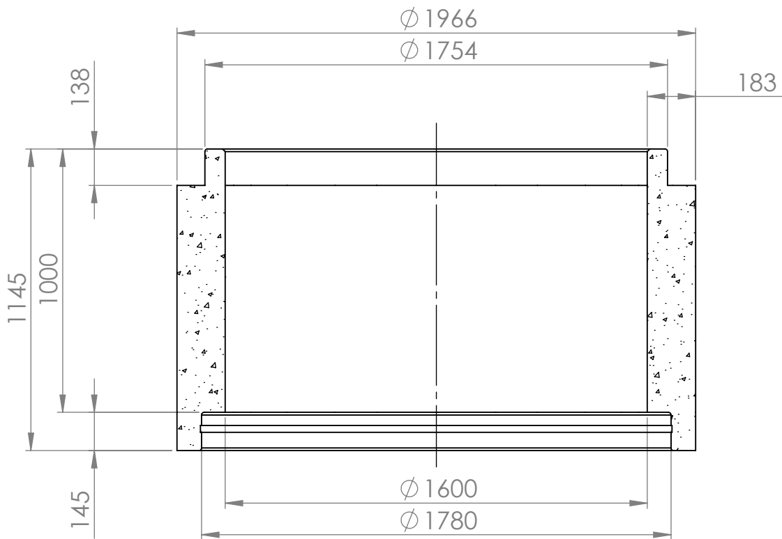
KESKILINJAN LEIKKAUS
