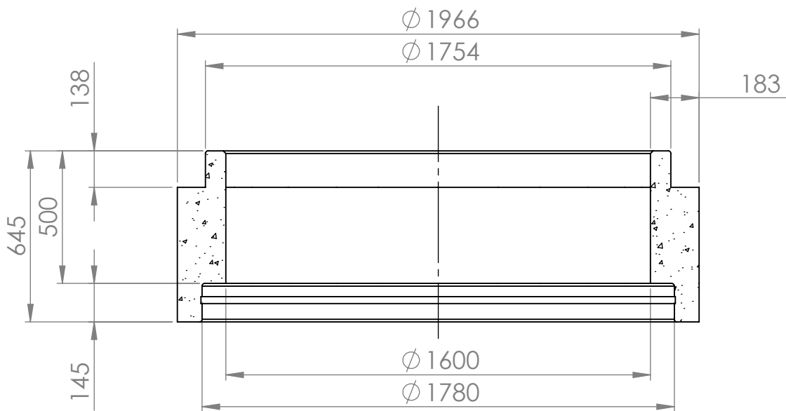
KESKILINJAN LEIKKAUS
