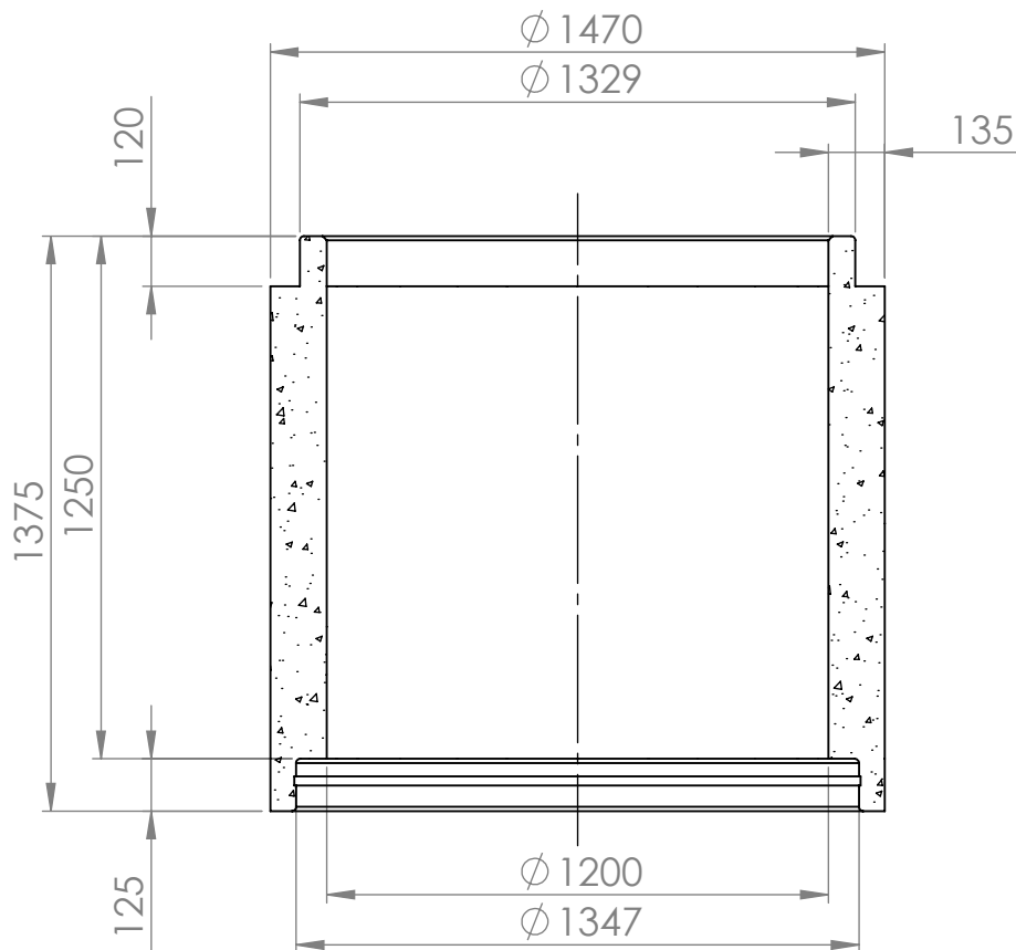
KESKILINJAN LEIKKAUS
