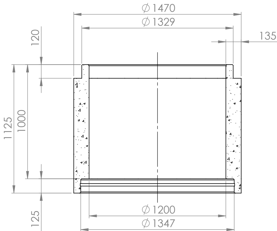
KESKILINJAN LEIKKAUS
