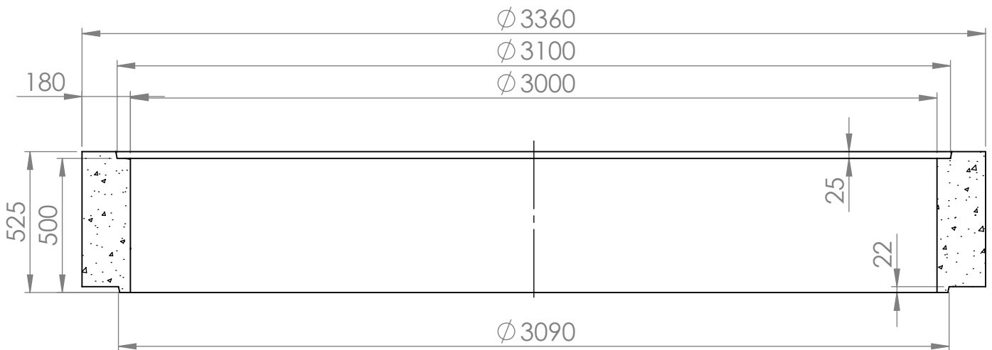
KESKILINJAN LEIKKAUS
