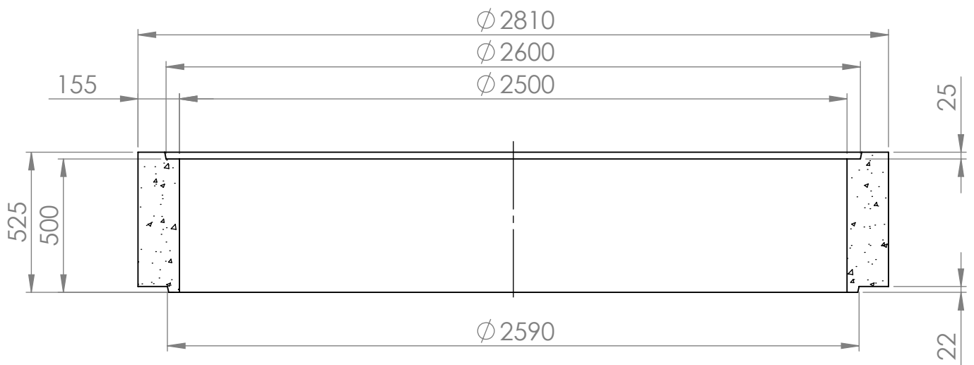
KESKILINJAN LEIKKAUS
