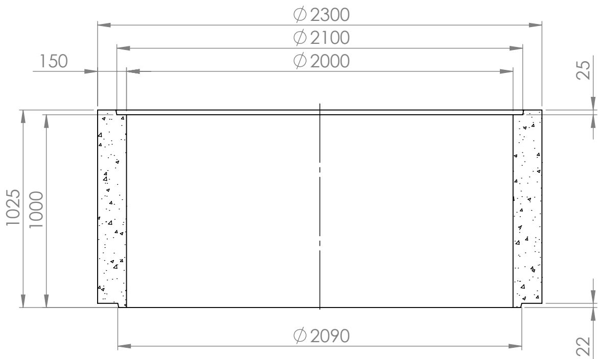
KESKILINJAN LEIKKAUS
