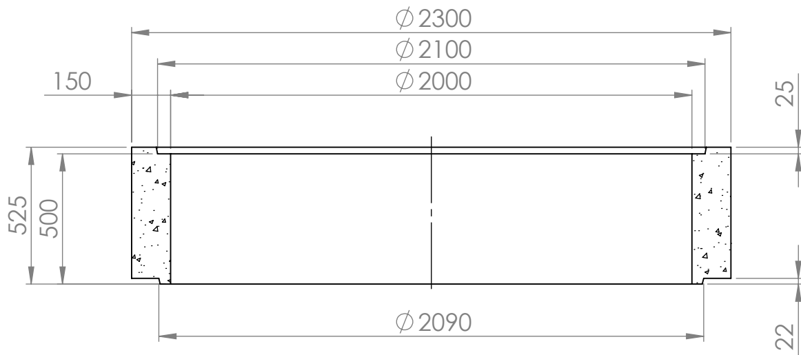
KESKILINJAN LEIKKAUS
